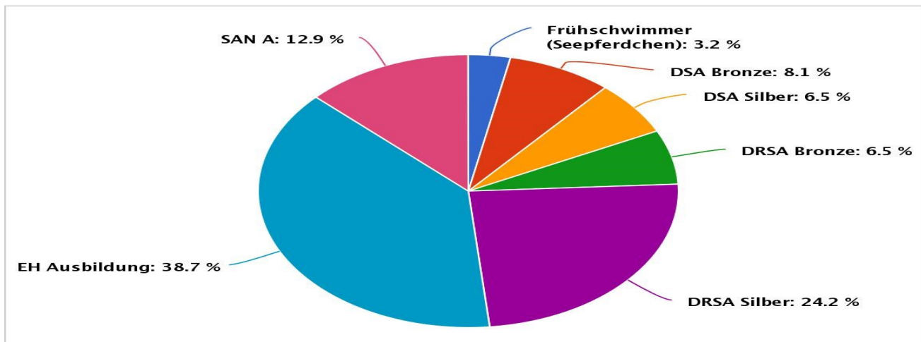
Statistik
